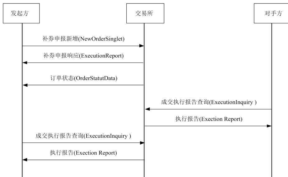
三方回购补券申报STEP消息流程
