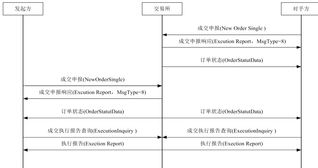
指定对手方报价STEP消息流程
