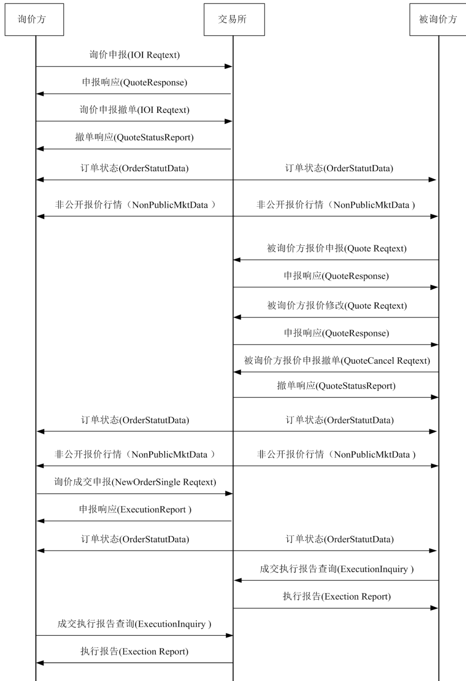
询价交易STEP消息流程
