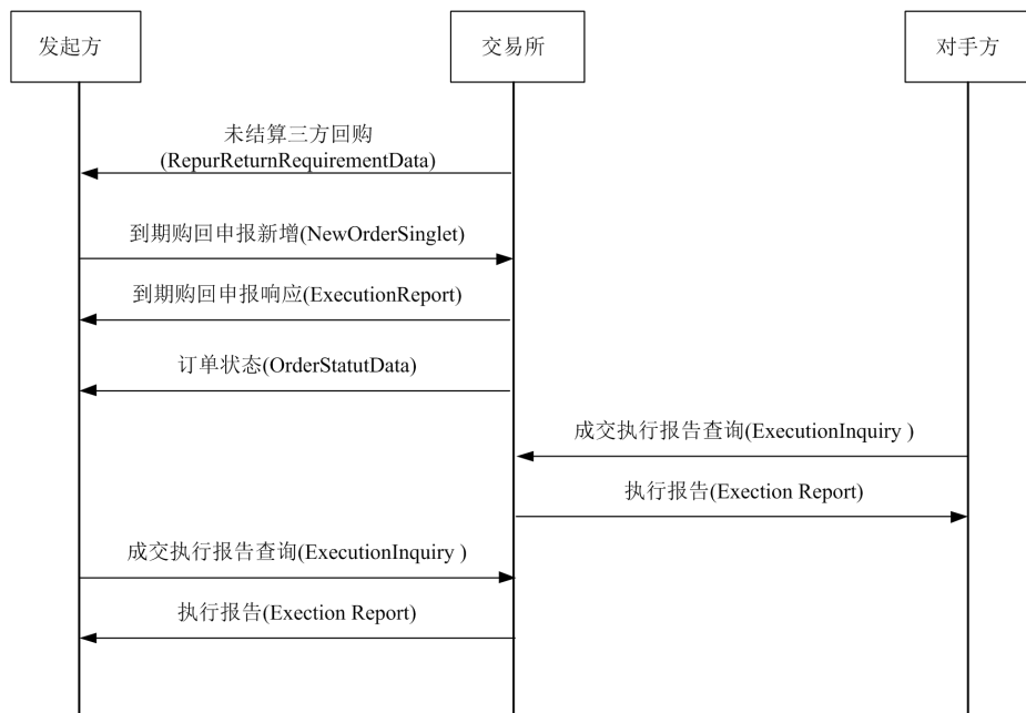
三方回购到期购回申报STEP消息流程
